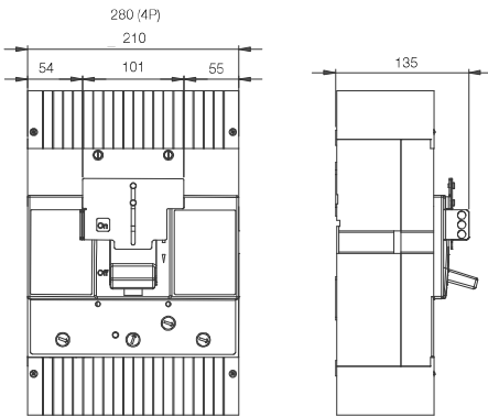
Mecánica 800-1000 + PLW800-1000
