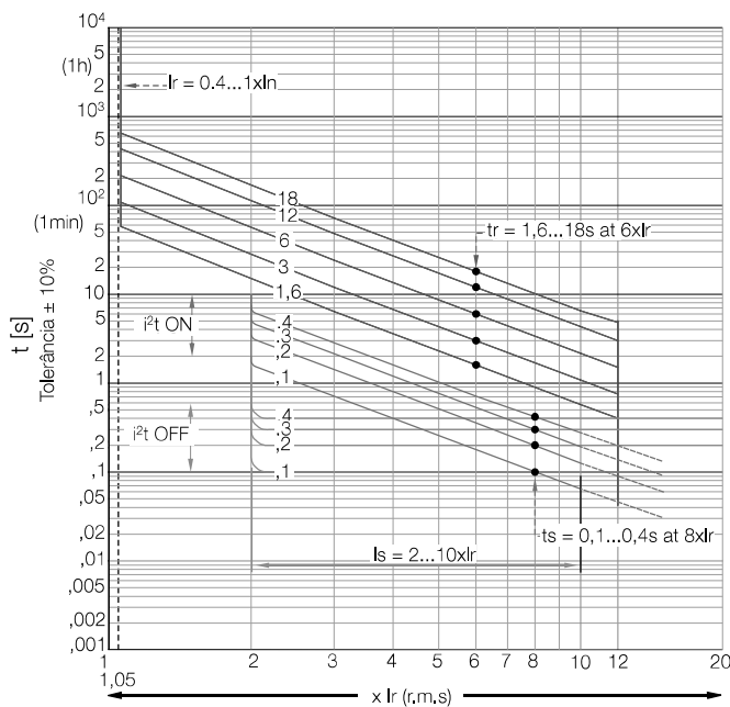
DWB1600 - Protección Contra Sobrecarga (L e S)
