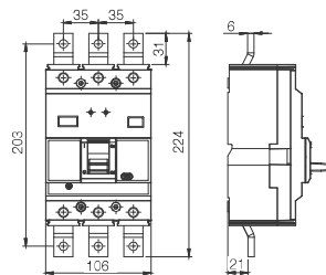
Mecánica 250 3P + BE DWB250 3P
