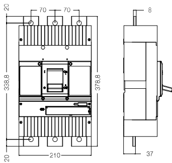
Mecánica DWB800-1000 3P + BE DWB800-1000
