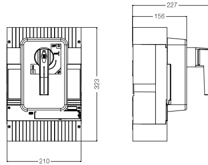
Mecánica 800-1000 3P + MRI DWB800-1000
