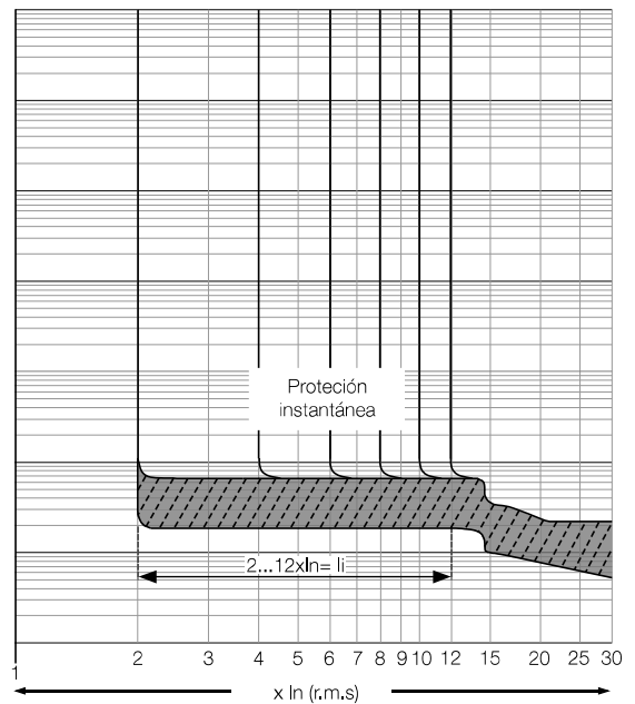
DWB1600 - Protección Contra Cortocircuito (I - Instantánea)
