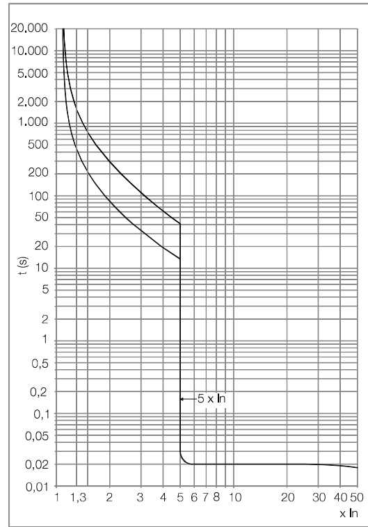
DWB250_G (Generador)
