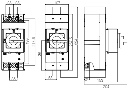
Mecánica 400 3P + MRI DWB400
