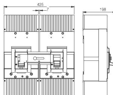
Mecánica 1600 3P + BLIM DWB1600
