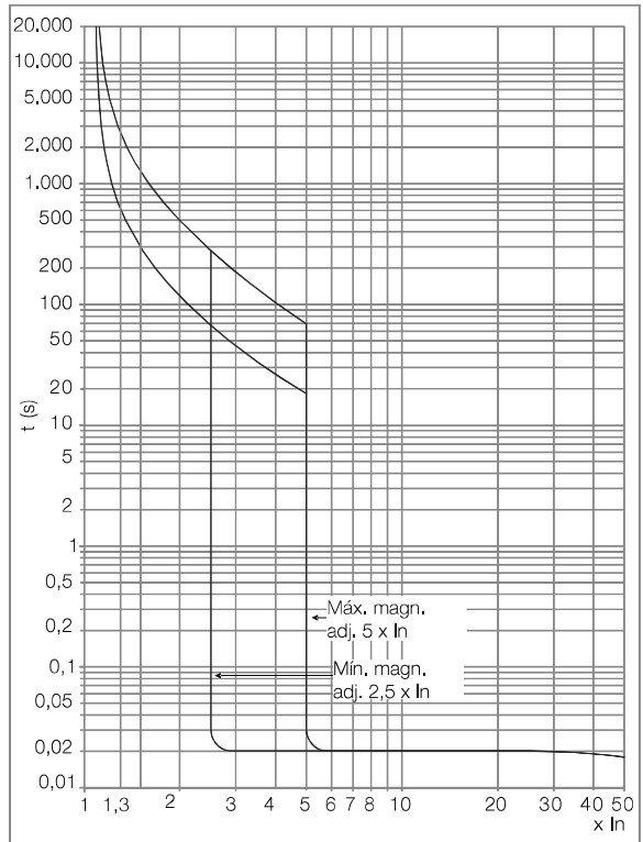
DWB800 (Generador)
