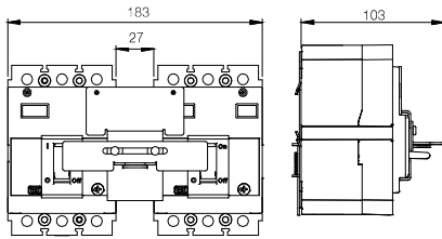
Mecánica 160 3P + BLIM DWB160 3P
