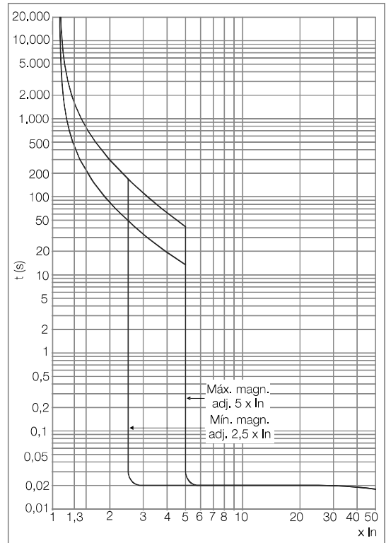
DWB400_G (Generador)
