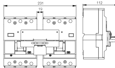
Mecánica 250 3P + BLIM DWB250 3P
