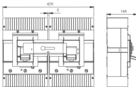
Mecánica 800 3P + BLIM DWB800 / DWB1000
