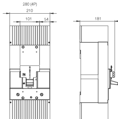
Mecánica 1600 + PLW1600
