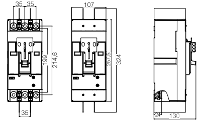
Mecánica 400 3P + PLW DWB400
