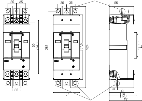
Mecánica 400 3P + BE DWB400 3P
