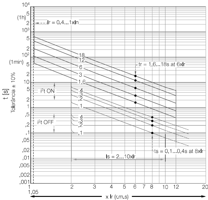
DWB1000 - Protección Contra Sobrecarga (L e S)
