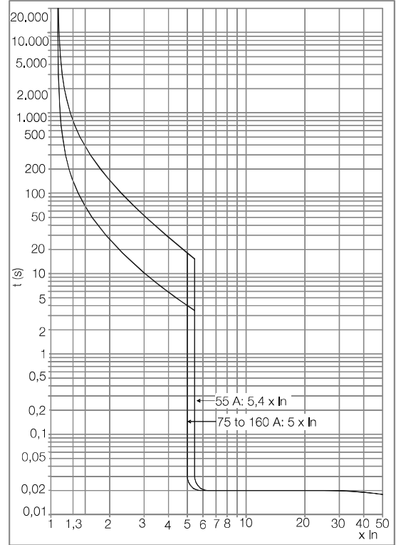
DWB160_G (Generador)
