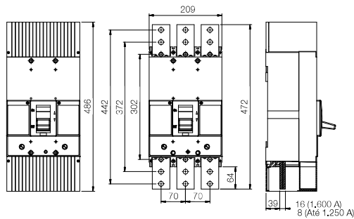
Mecánica 1600 3P + BE DWB1600
