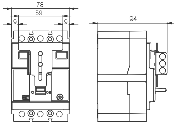
Mecánica 800-1000 + PLW800-1000
