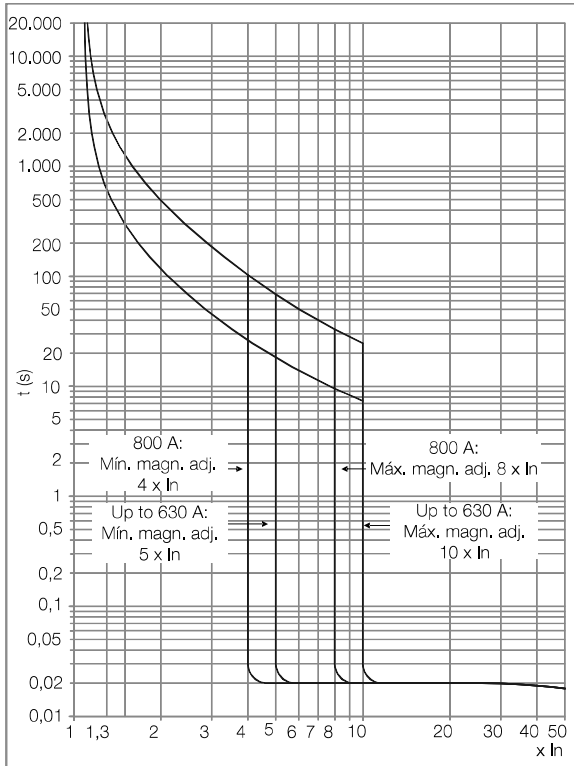
DWB800 (Distribución)
